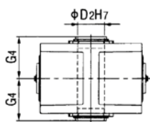
P3HV 空心轴 Hollow shaft
