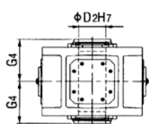
P2HV 空心轴 Hollow shaft
